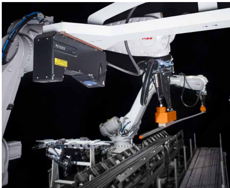
Stabentnahme mit einem Magnetgreifer durch KASTOpick bar
